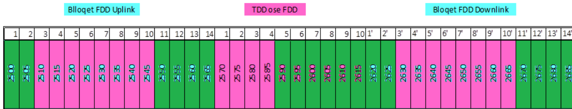
Spektri i çiftuar bllloqet 1-14 FDD Uplink me bllloqet 1'-14' FDD downlink Spektri i paciftuar bllloqet 1-10 TDD ose FDD
