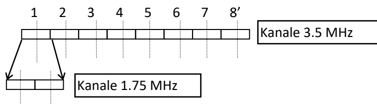
(b) Nën-ndarja e mëtejshme në kanale me gjerësi 1.75 MHz
