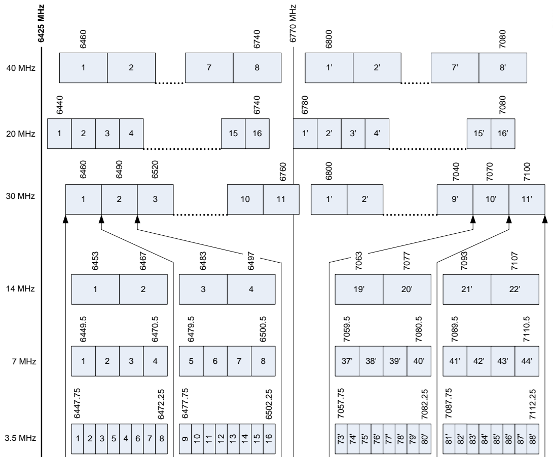
Figura 8. Ndarja e kanaleve për brezin 6425 – 7125 MHz
